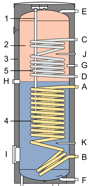
Schnittdarstellung des WW 300-S
